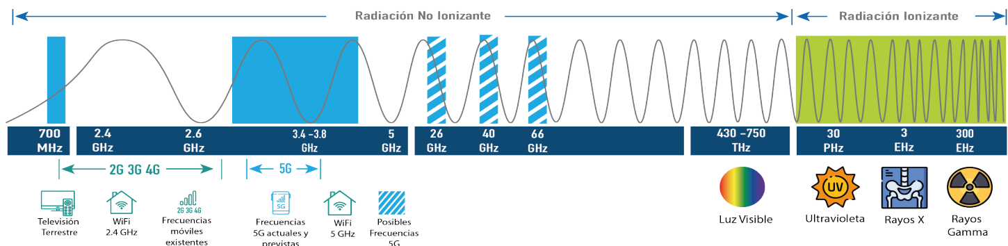
FIGURA 1: ESPECTRO ELÉCTROMAGNÉTICO
